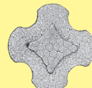
车削针4点形横截面
