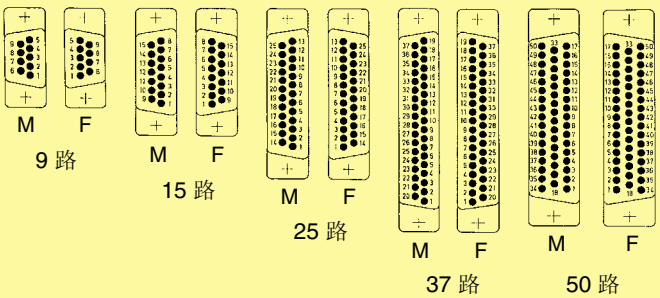
针布置 连接侧视图
